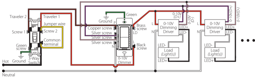
Wiring Scheme 1
