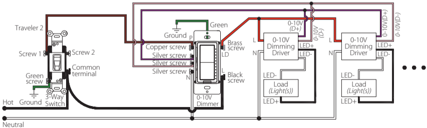
Wiring Scheme 2
