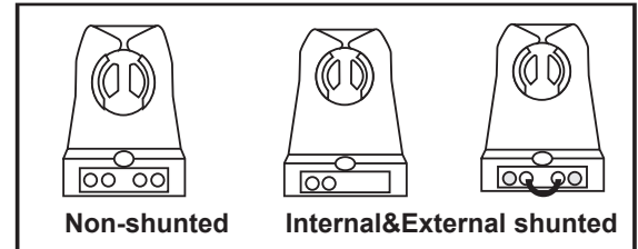
Fig:1 -Lampholder Type
