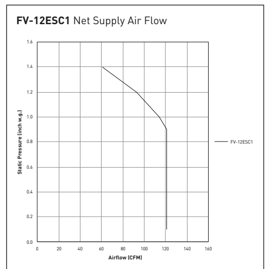
FV-12ESC1
