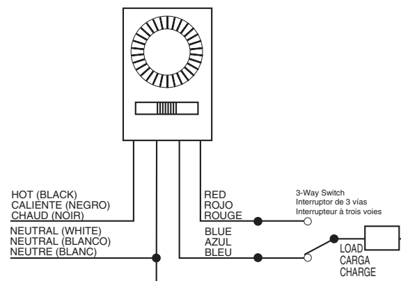
3-Way Installation/Instalación de 3 vías/Installation à trois voies
