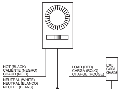
Standard Installation/Instalación estándar/Installation normale
