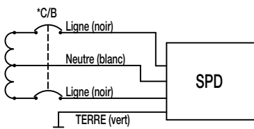
SCHEMAS DE CÂBLAGE DES SPD DE TYPE 2 120/240 VCA MONOPHASÉ
