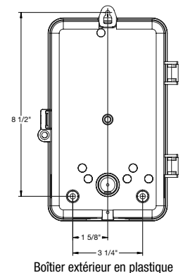
Boîtier extérieur en plastique
